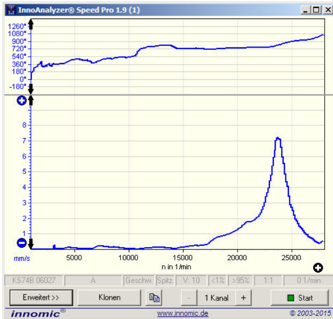
Betrag und Phase für frei einstellbare Ordnungen
